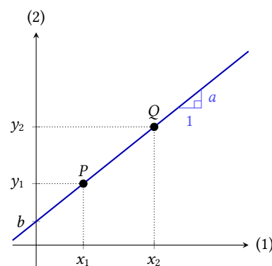
Figur 6.2: De to punkter P og Q på grafen for f(x) = a \cdot x + b .
