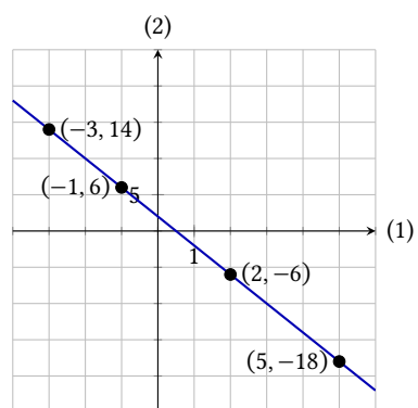
Figur 5.4: Data fra tabel 5.2 indsat i et koordinatsystem. Grafen er herefter tegnet ud fra punkterne.
