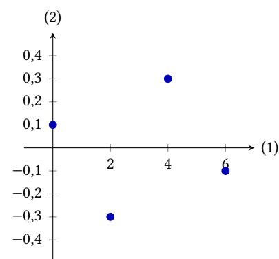
Figur 7.5: Residualplot over værdierne i tabel 7.4.
