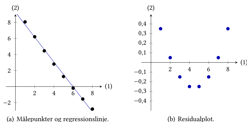
Figur 7.6: En række målepunkter med regressionslinje samt residualplottet. Regressionslinjen ser ud til at passe godt på målepunkterne, men residualplottet afslører at modellen faktisk ikke passer ret godt.
