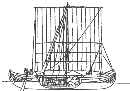
a) Havgående handelsskib (måske kildernes »knarre«). Mål: 16,3 \times 4,5 m Lasteevne: 15-20 tons Bemanning: ukendt – måske kun 5-6 mand.
