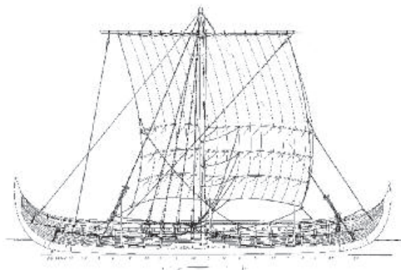
Sejlplan af Gokstadskibet
