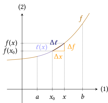
Figur 4.2: \Delta\ell er næsten lig med den lille trekants hypotenuse.
