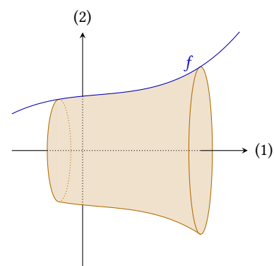
Figur 4.4: Omdrejningslegemet for grafen for en funktion f .
