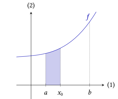
Figur 3.2: A(x_0) svarer til det viste areal.
