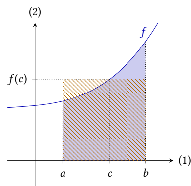
Figur 4.1: Arealet under grafen svarer til arealet af det skraverede rektangel.
