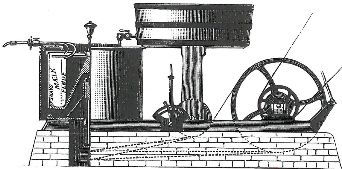
Centrifuge fra Maglekilde ved Roskilde fra 1878. Ved at sætte en beholder til at dreje rundt blev mælken delt. Skummetmælken blev slynget ud mod kanten, mens fløden blev liggende i midten. Inden centrifugen havde man måttet vente på, at mælken selv skiltes. Centrifugen kunne drives af en hestegang, men det blev normalt at koble den til en dampmaskine, der også kunne drive smørkernen.
