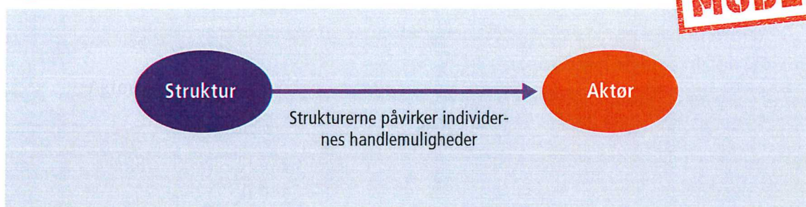
Figur 1.3 Deterministisk perspektiv
