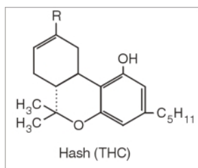
Fig. 4.1. Den kemiske grundformel for hash. Ved R kan der sidde forskellige funktionelle grupper, som dermed ændrer stoffets kemiske egenskaber.
