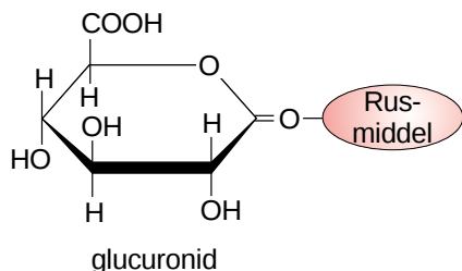
Fig. 2.7. Glucuronidsyrens molekylestruktur. Glucuronid dannes i organismen ud fra glucose.
