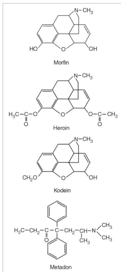
Fig. 7.1. De vigtigste opioiders molekylstruktur.
