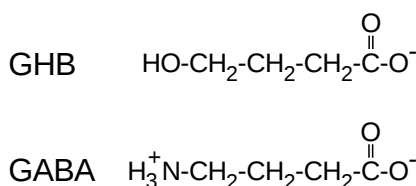
Fig. 6.1. GHB's molekyleformel ses at minde meget om GABA.
