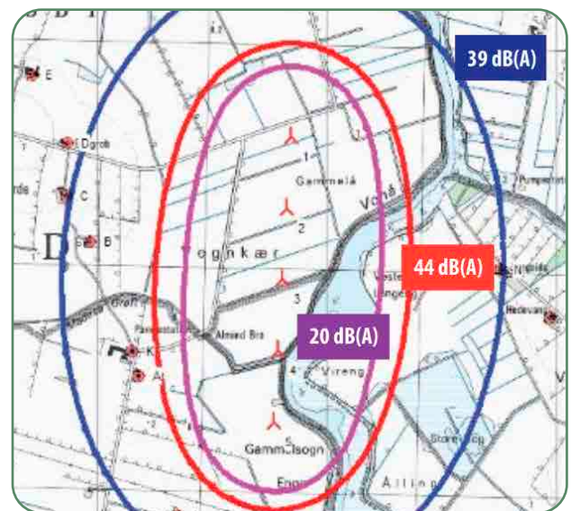
Kort med støjgrænser for vindmøllepark
