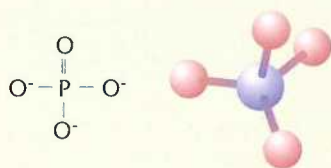
Figur 40. Den rumlige struktur af fosfat, \text{PO}_4^{3-} .
