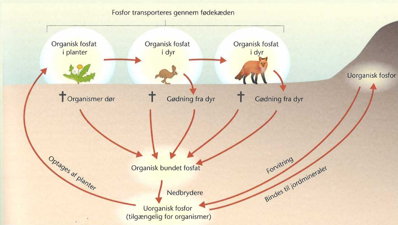
Figur 39. Det globale fosforkredsløb.
