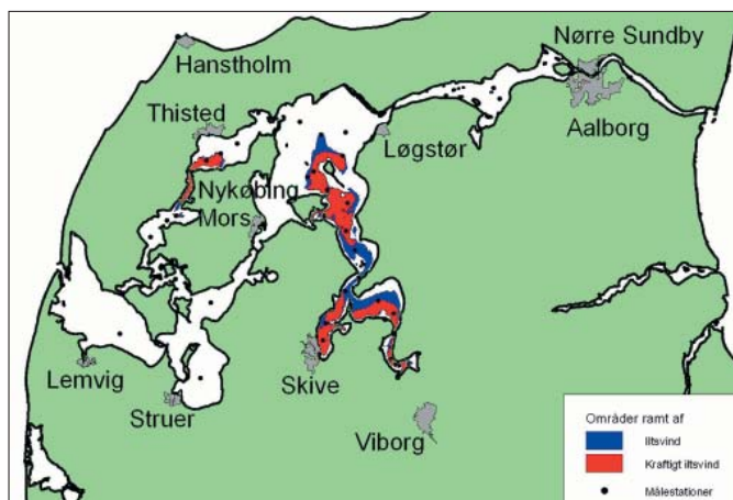
Figur 7. Omfattende og tidligt iltsvind i Limfjorden 2007. I alt var godt 13% af fjorden areal ramt af iltsvind, heraf godt 8% med kraftigt iltsvind med iltindhold på under 2 mg/l (rødt område) i uge 24.
