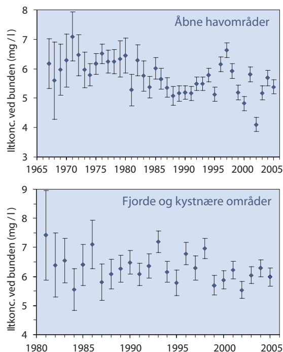
Figur 2: Middelmiddelt koncentration af ilt (juli-november) i bundvandet for stationer i åbne havområder samt fjorde og kystnære områder. Kilde: Ærtebjerg et al., 2005.
