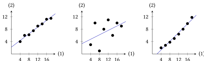
Figur 6.8: Tre eksempler på lineær regression. Kun på den første figur virker en lineær model rimelig.
