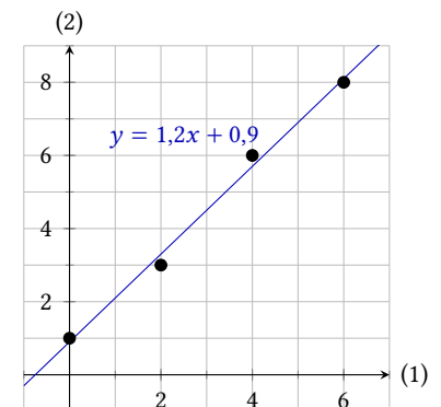
Figur 6.7: Den bedste rette linje gennem de 4 punkter.
