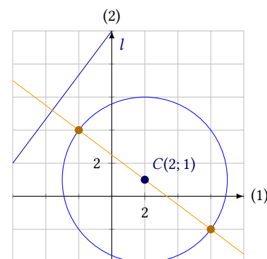
Figur 6.5: Røringspunkterne for de cirkeltangenter, der er parallelle med linjen l .
