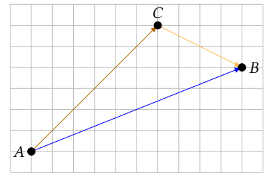
Figur 1.10: Indskudssætningen: \overrightarrow{AB} = \overrightarrow{AC} + \overrightarrow{CB} .
